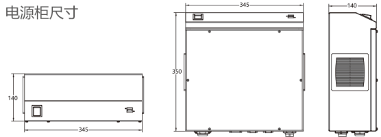
电源柜尺寸
