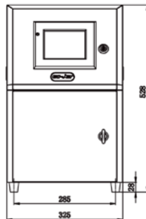
EC-JET1000尺寸示意图 单位: mm
