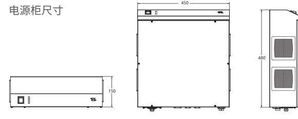
电源柜尺寸
