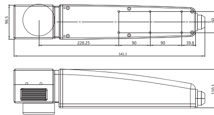
打标单元尺寸
