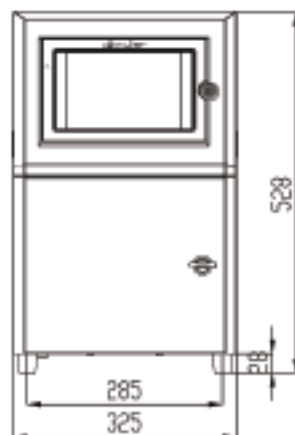
EC-JET1000Pro尺寸示意图 单位:mm
